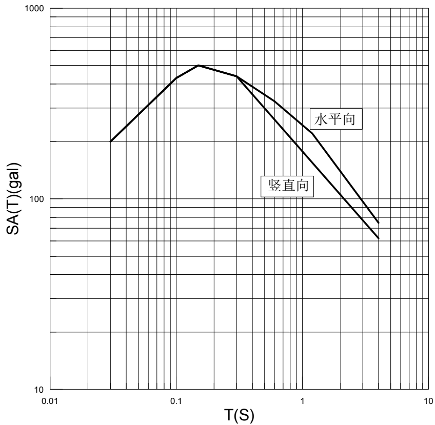
附图 厂址特定 SL-2 级地面运动基岩加速度反应谱 (5%阻尼比)
